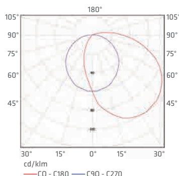
OPTIMA 1 2x9W
