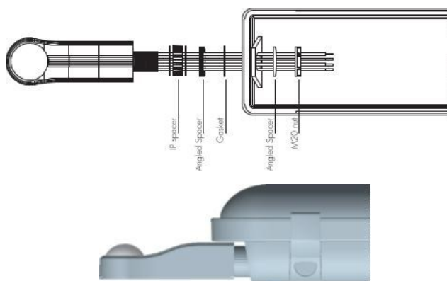
Typowa instalacja 2
