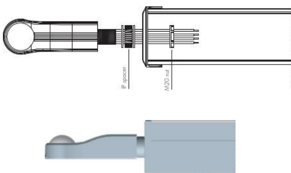
Sposób instalacji 1
