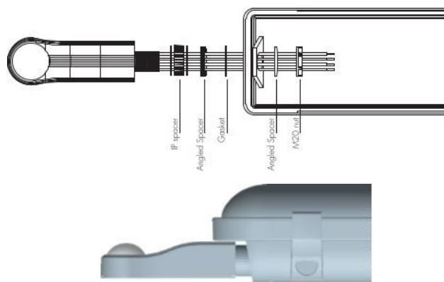
Sposób instalacji 2
