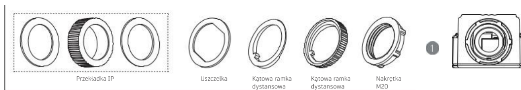
Sposób instalacji 2
